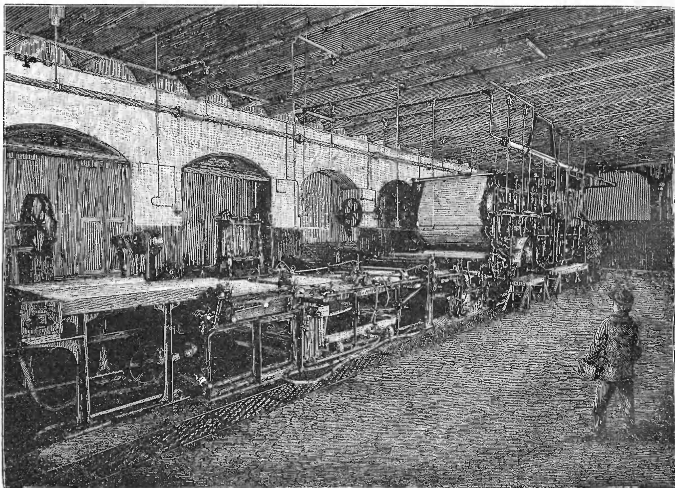
Эксп. Загот. Госуд. Бумагъ въ СПб. Большая бумагодѣлательная машина. По фотогр. грав. М. Рашевскій.
